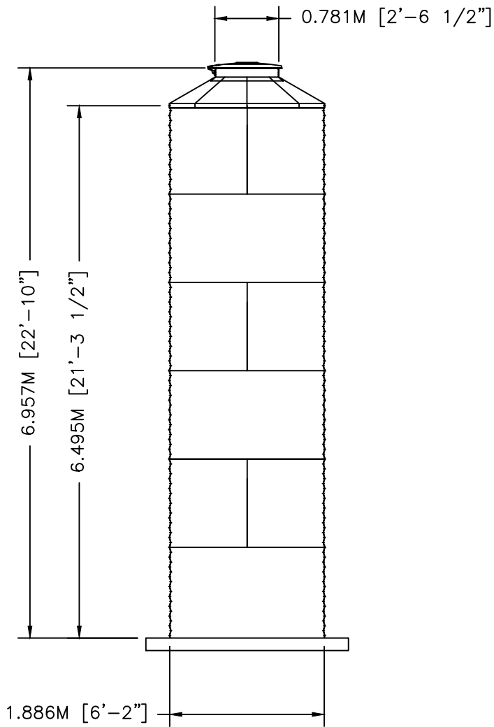
ELEVATION
